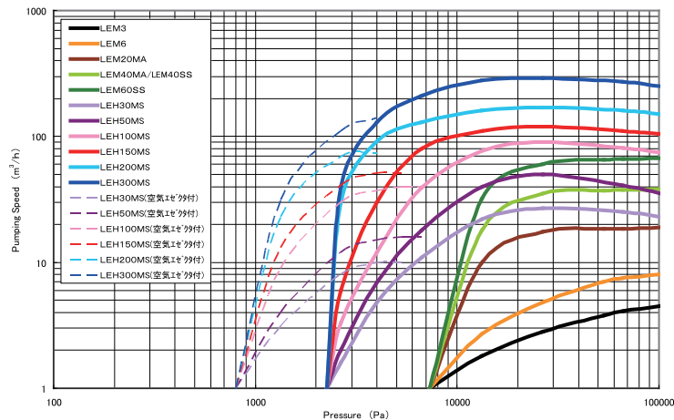
水封ポンプ性能グラフ（周波数60HZ、給水温度15℃）
