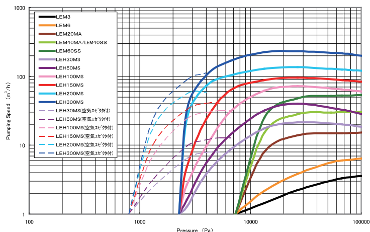
水封ポンプ性能グラフ（周波数50HZ、給水温度15℃）
